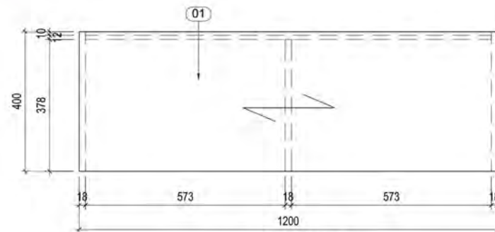
MẶT BẰNG TL:1/10
