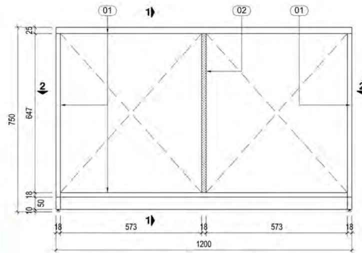
MẶT ĐỨNG TL:1/10
