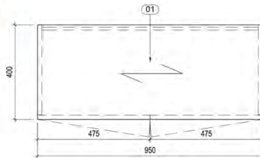
MẶT BẰNG TL:1/10
