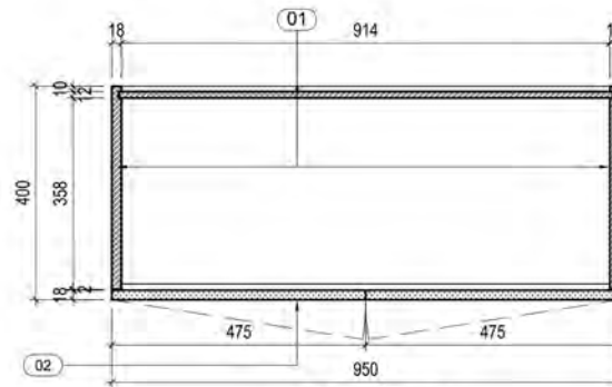
MẶT CẮT 2-2 TL:1/10
