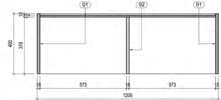
MẶT CẮT 2-2 TL:1/10
